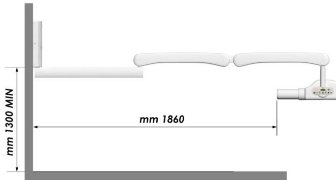
Wandbefestigung mit Querarmlänge 80 cm
