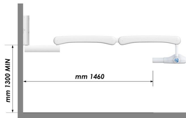
Wandbefestigung mit Querarmlänge 40 cm
