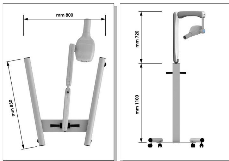
Ansicht und Abmessungen fahrbare Version
